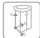
Зеркало SMART с выдвижным механизмом A - 500 мм B - 650 мм C - 120 мм
